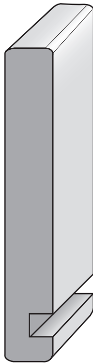
PAC 3131 1/2 X 3-1/4
